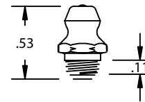
1/4"-28 TAPER THD. (SAE-LT)
