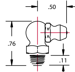
1/4"-28 TAPER THD. (SAE-LT)
